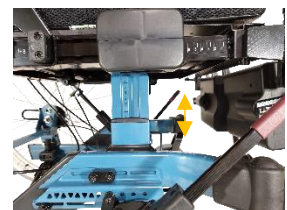
Verstellung um 70 mm mit Hilfe des Adapters
